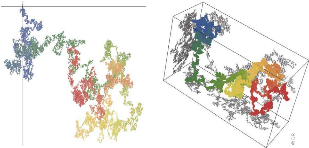
Des marches aléatoires de 20 000 pas approximant le mouvement brownien en dimensions 2 et 3. À droite, les projections orthogonales de la trace brownienne sont représentées sur les faces de la boîte.
