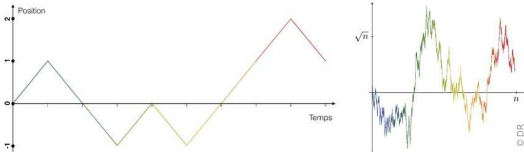
Une marche aléatoire de 9 pas (à gauche) et une marche aléatoire de 20 000 pas (à droite). La couleur de la particule évolue du bleu au rouge au cours du temps. Dans la figure de droite, une courbe aléatoire très irrégulière apparaît : c'est le mouvement brownien en dimension 1.
